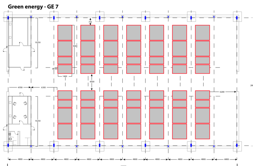
Ustawienie generatorów i wymiary Bezemisyjnej Siłowni Energetycznej Green Energy - GE 7MW
